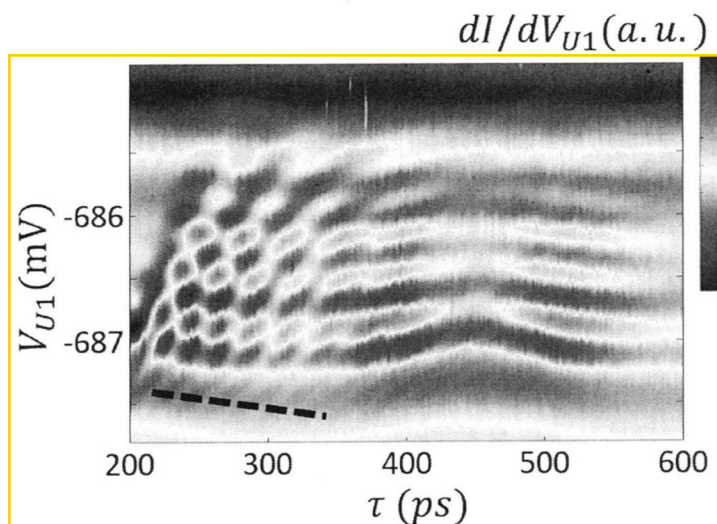
图 3.8 实验中测得的 OPC 微分电导随电压 V_{U1} 和自由演化时间 t_p 的关系。
