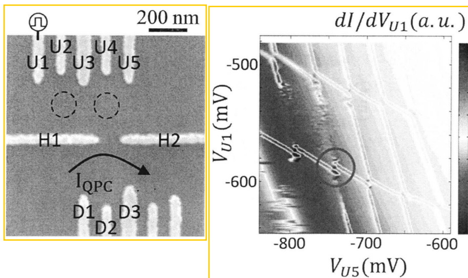
图 3.2 (1) 实验制备的 GaAs/AlGaAs 双量子点样品结构图。(2) 利用 OPC 锁相调制技术测量得到的电荷稳态分布图。
