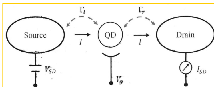
图 1.3 单量子点结构示意图， \Gamma_l 、 \Gamma_r 分别为量子点与源漏间电子隧穿率， V_g 为量子点栅电极电压。
