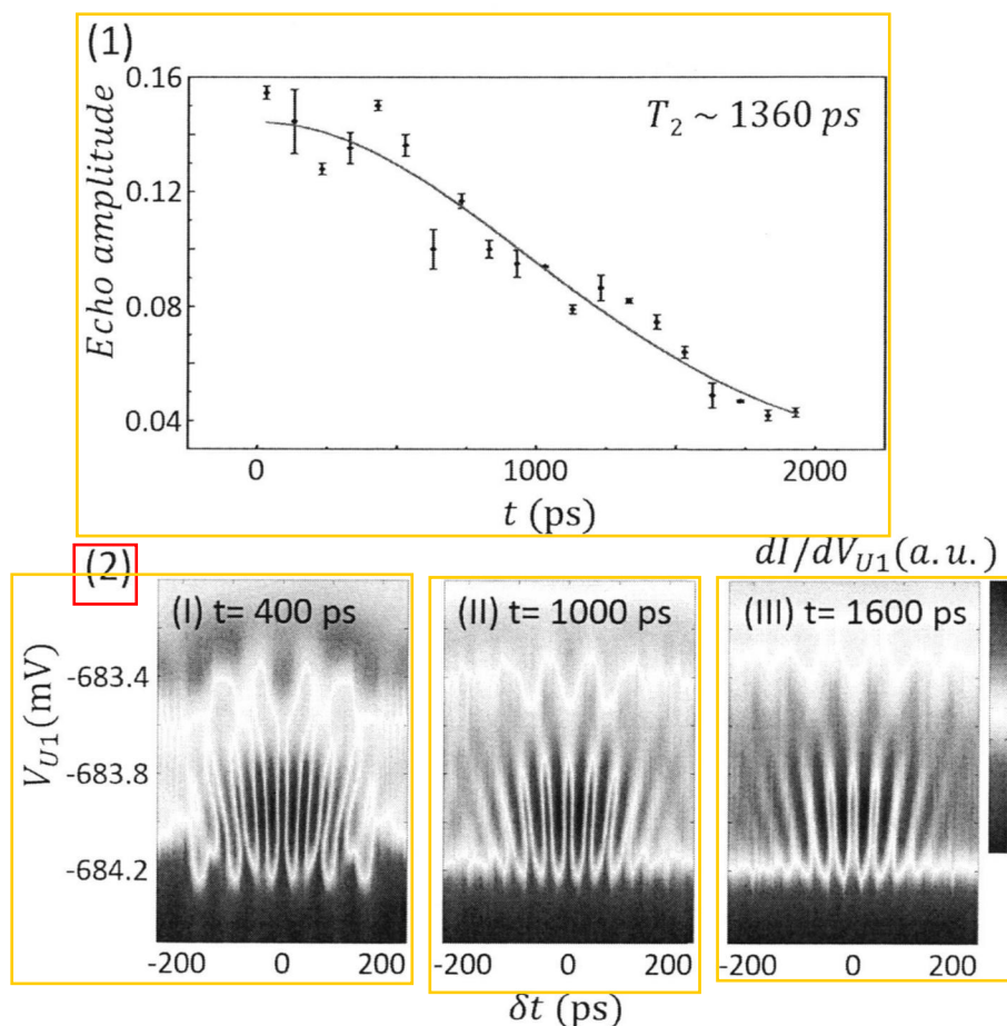
图 3.12 (1) 从实验结果提取的回声幅度随总演化时间 t 的变化关系，从中拟合出非均匀消相干时间 T_2 = 1360 \pm 400 ps。(2) 利用实验数据模拟得到的回声过程。
