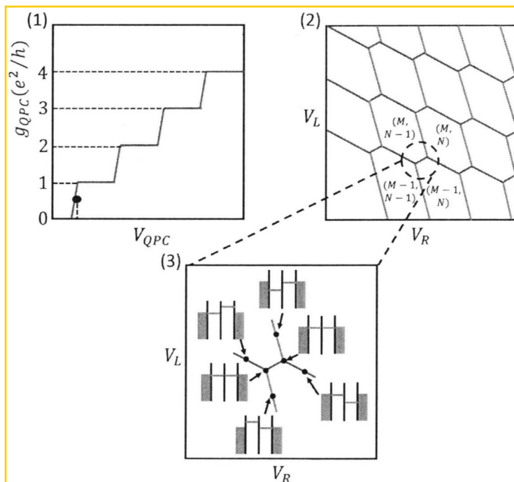
图 1.8 双量子点电荷感应测量结果。(1)QPC 量子化电导示意图，黑点为 QPC 工作时所在的位置。(2)QPC 测量得到的电荷稳态分布图，每条充电线对应一个 QPC 微分电导峰。(3) 双量子点充电线反交叉区域对应的电势关系。
