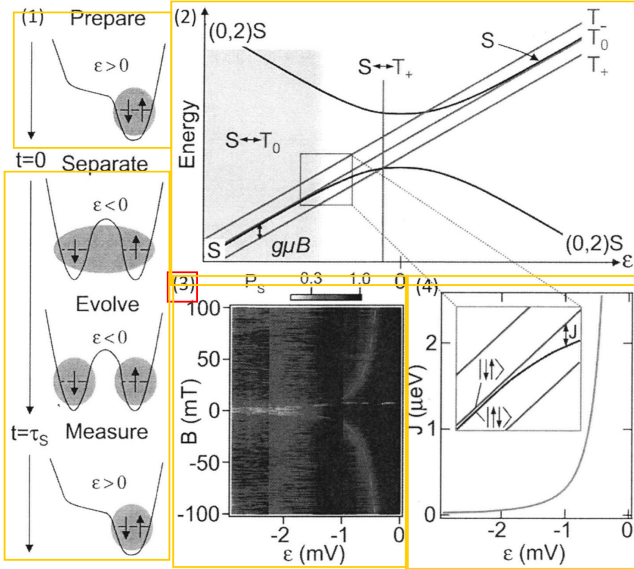
图 2.4 (1) 对双量子点 S-T_0 态进行操控时电子态变化示意图。(2) 在外加磁场作用 B_z 下 (1,1)-(0,2) 反交叉区域能级示意图。(3) 实验测量得到的 S-T_0 交叉点所在位置随外磁场变化关系。(4) S-T_0 交换相互作用 J 的大小随失谐量 \epsilon 的变化关系。(图片引自文献 [32])
