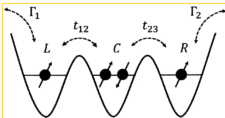
图 5.1 线性耦合的三量子点结构示意图。
