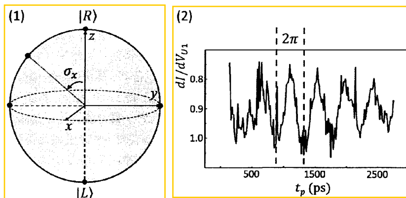
图 3.5 (1) Bloch 球上 \sigma_x 操作示意图。(2) 图 3.4.2 中红色虚线处截取的 Larmor 振荡曲线, 每个峰间隔表示比特状态在 Bloch 球上绕 x 轴转动一周。
