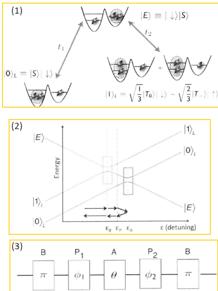
图 4.2 (1) 双量子点中占据三个电子能级示意图。(2) 模拟计算所得的三能级结构示意图。(3) 完成一个比特任意操作所需过程示意图。(图片引自文献 [36])
