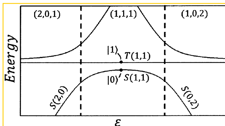
图 6.3 简化后的 exchange qubit 能级结构。
