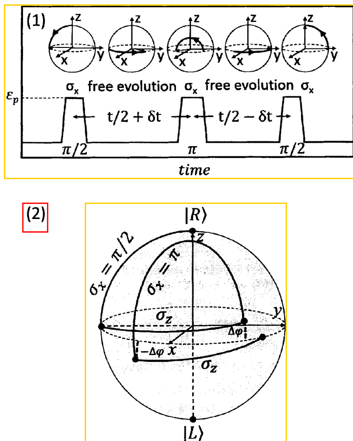
图 3.10 (1)charge echo 所采用的非绝热脉冲示意图以及对应的比特状态在 Bloch 球上演化过程。(2)echo 翻转消除噪声扰动的一种直观理解, 两次 \sigma_x 转动过程中产生的轨迹偏移量 \Delta\phi 相互抵消。
