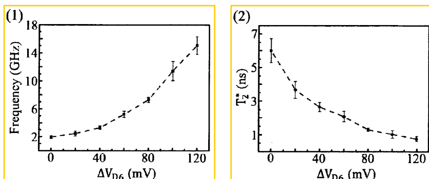
图 6.7 (1) 实验测得的 Larmor 振荡频率随电压 V_{D6} 的变化关系。(2) 从系列相图中虚线位置提取振荡曲线, 拟合得到的相干时间 T_2^* 随电压 V_{D6} 的变化关系。
