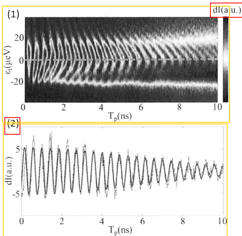
图 4.6 (1) 实验得到的 Larmor 振荡相图。(2) 从 (1) 图中虚线处提取的振荡曲线，通过拟合得到相干时间 T_2^* = 8.1\text{ns} 。
