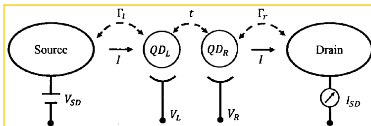
图 1.5 串联双量子点结构示意图, t 为量子点间的隧穿耦合强度。
