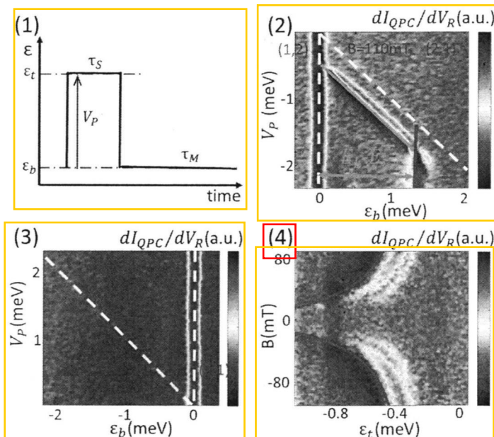
图 2.7 (1) 用来观察自旋阻塞效应的脉冲波形示意图。(2) 脉冲向负失谐量方向施加时测量得到的三电子态隧穿相图。(3) 脉冲向正失谐量方向施加时的隧穿相图。(4) 测量所得 OPC 微分电导随外加磁场和脉冲高度的变化关系，从中可以拟合出 J_s 。
