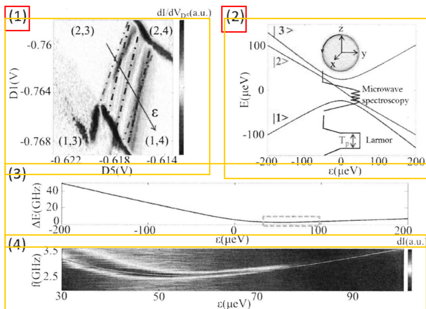
图 4.5 (1) 通过在电极 D5 施加电压短脉冲后得到的 (1,4)-(2,3) 电子隧穿相图。(2) 模拟得到的能级结构图。(3) 计算所得 |1> 和 |2> 态能级间隔。(4) 利用微波共振技术从实验上测得的 |1> 和 |2> 能级间隔。
