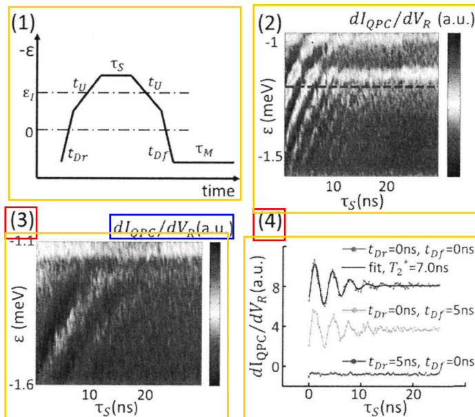
图 2.8 (1) 用来实现 LZS 过程采用的脉冲示意图。(2)、(3) 不同外加磁场大小下的 LZS 干涉。(4) 不同上升沿时间下的 (2) 中虚线所示位置的振荡曲线。
