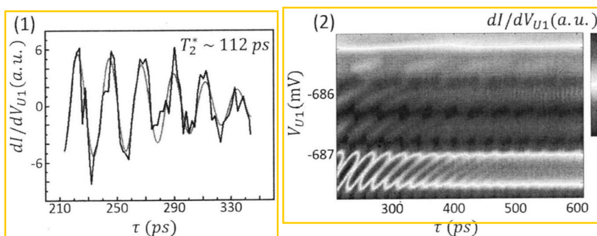
图 3.8 实验中测得的 OPC 微分电导随电压 V_{U1} 和自由演化时间 t_p 的关系。
