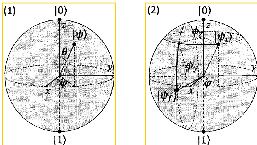
图 1.1 (1) 描述量子比特状态的 Bloch 球示意图, |0\rangle 和 |1\rangle 为量子比特基态, |\psi\rangle 为任意叠加态; (2) 实现单个比特任意操控示意图, 比特初始态为 |\psi_i\rangle , 经过 \phi_z 和 \phi_y 两次旋转到达任意末态 |\psi_f\rangle 。
